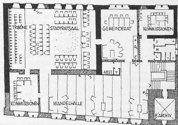
1. OBERGESCHOSS
