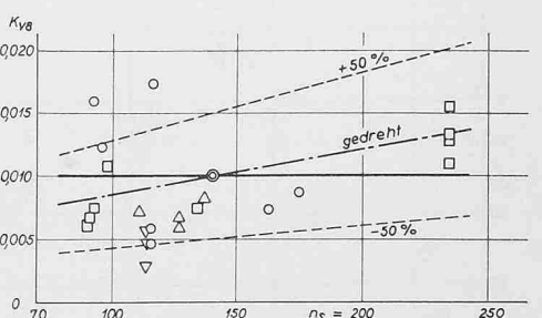
Bild 25. Koeffizienten K_{v8} der Formel nach Abschnitt 4.3.8 in Abhängigkeit von der relativen Radbreite B/D bzw. von der spezifischen Drehzahl n_s .
