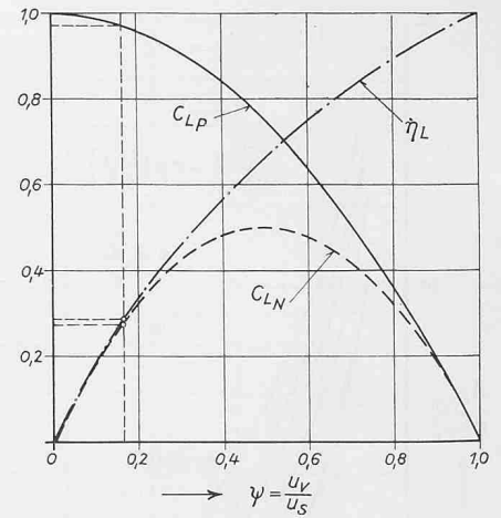
Bild 6 (rechts). Pumpenleistungsziffer C_{LP} , Nutzleistungsziffer C_{LN} und Wirkungsgrad \eta_L im Lüftungsabschnitt. Daten des gestrichelt eingezeichneten Beispiels: u_s = 30 \text{ m/s} ; u_v = 5 \text{ m/s} ; \Psi = 0,167 ; C_{LP} = 0,97 ; C_{LN} = 0,27 ; \eta_L = 0,286
