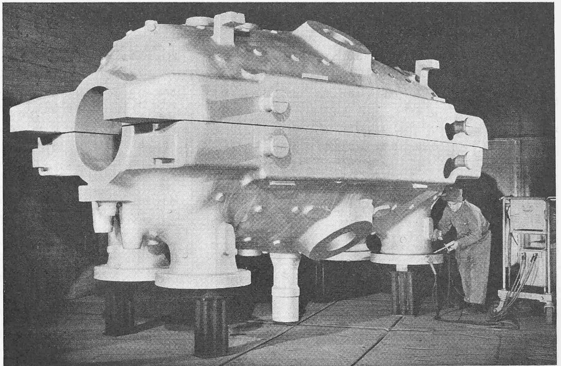
Bild 4 (Mitte). Hochdruck-Dampfturbinen-Innenzylinder aus 11% Cr-Stahlguss (VIS 11). Gewicht 13,5 t. Geliefert an Siemens-Schuckertwerke AG, Mülheim-Ruhr. Deutschl.
