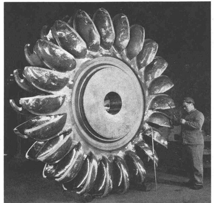
Bild 1 Verschleiss- und korrosionsbeständiges Laufrad einer siebenstufigen Hochdruckpumpe, gegossen im Präzisionsgussverfahren aus einer hochlegierten martensitischen Chromkobaltlegierung.
