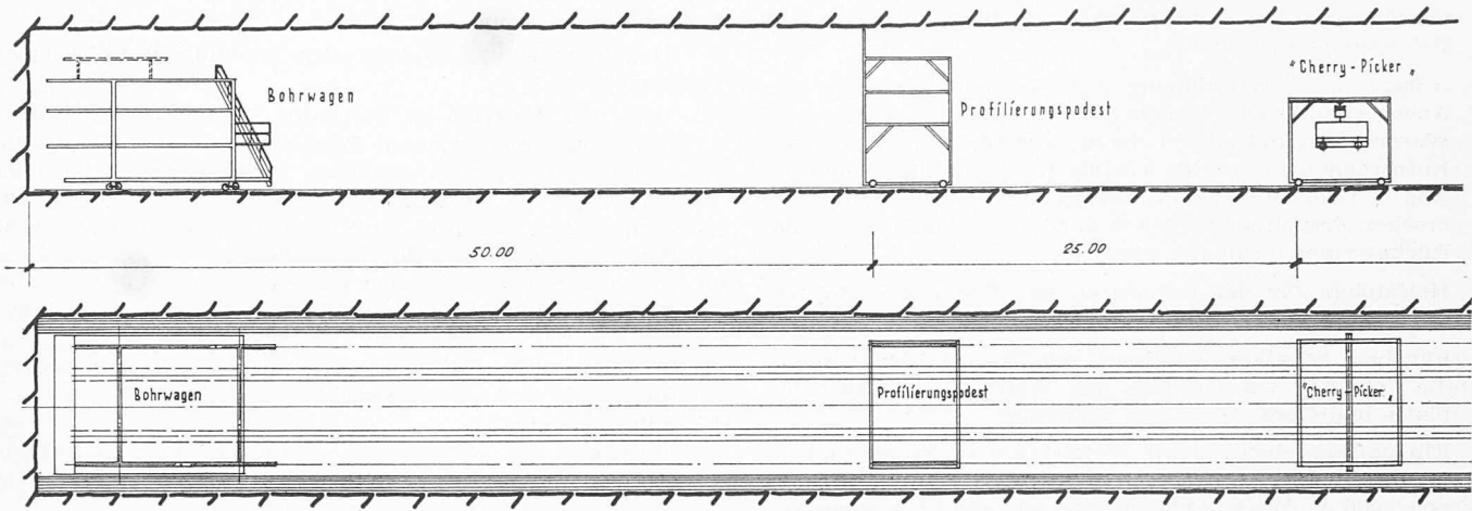
Bilder 2 und 3. Bohren, Längsschnitt und Grundriss, Masstab 1:500
