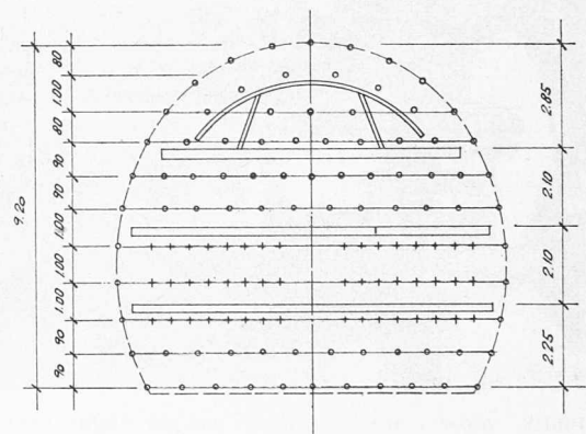
Bild 6. Schnitt A-A zu Bild 4 und 5
