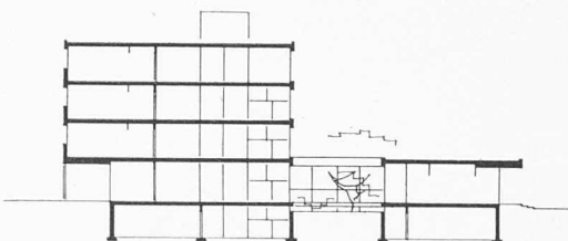
Schnitt Südwest—Nordost 1:600
