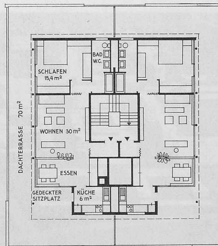
Attikageschoss der Turmbauten, 1:300
