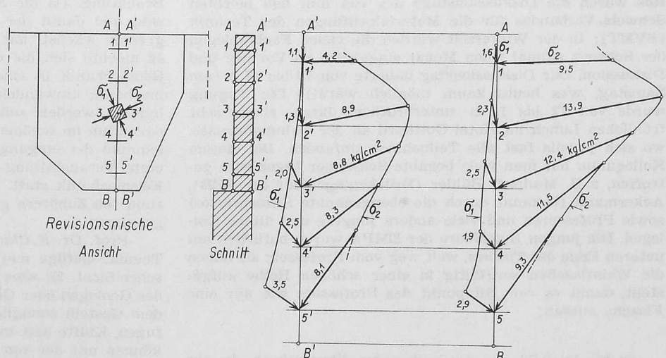
Bild 33. Modell M 2 ; Spannungsverlauf längs eines Vertikalschnittes durch die Wand der Revisionsnische
