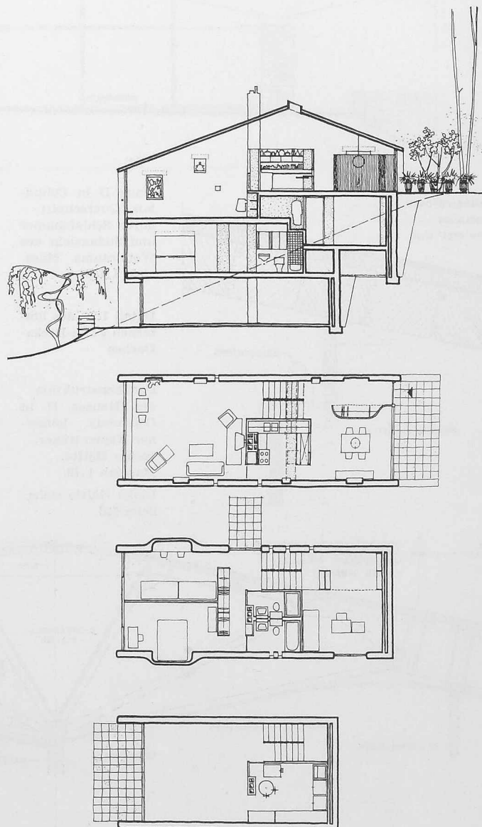
Haus am Steilhang, Grundrisse und Schnitt 1:250
