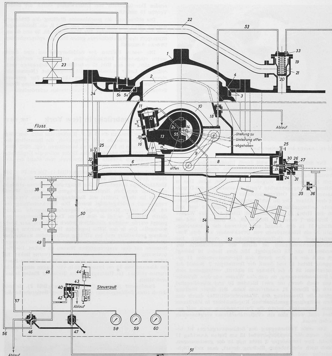
Bild 12. Schema der Schieberbetätigung
