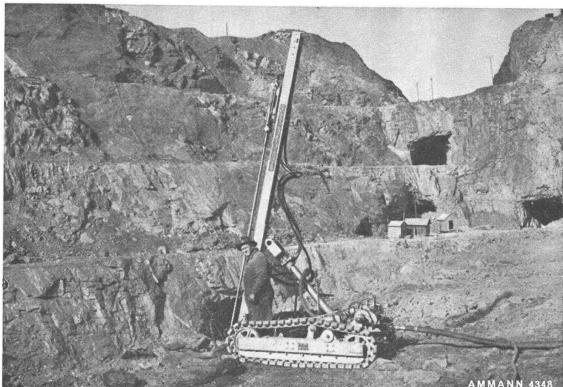
Raupen-Bohr-Fahrzeug «Air-Trac»
