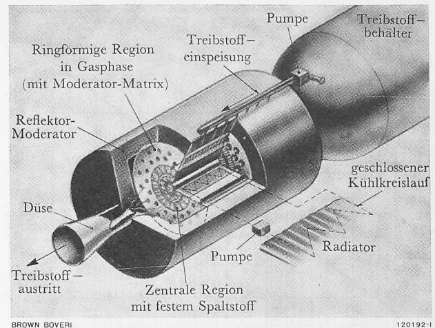
Bild 9. Vorschlag für einen fortgeschrittenen Raketen-Reaktor in Zweizonen-Ausführung nach [3]. Die zentrale Zone (mit geschlossenem Kühlkreislauf) enthält feste Brennstoffelemente, in der periphenen Zone nimmt gasförmiger Spaltstoff mit Wasserstoffgas vermischt an der Kettenreaktion teil und erhitzt den Wasserstoff direkt durch Übertragung der kinetischen Energie der Spaltfragmente auf hohe Temperaturen.
