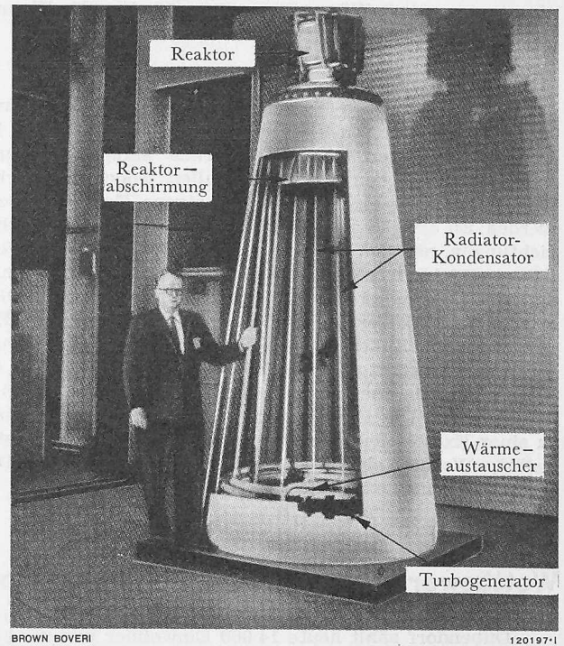
Bild 14. SNAP-2-Reaktorsystem, komplett, nach [3]. Die Reaktorleistung beträgt 50 kW th , die elektrische Nettoleistung nur 3 kW. Für den Primärkreislauf wird NaK, für den Sekundärkreislauf Hg verwendet.
