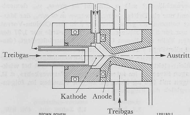
Bild 10. Elektrothermischer Antrieb (Lichtbogen-Jet), nach [4]
