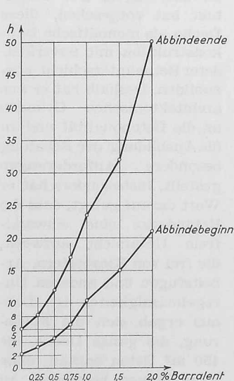
Bild 1. Verzögerung der Betonabbindezeit bei Beton mit Zement Liesberg PC 300 bei einer Lufttemperatur von 18 bis 20^\circ \text{C} durch die Beimischung von Barralent
