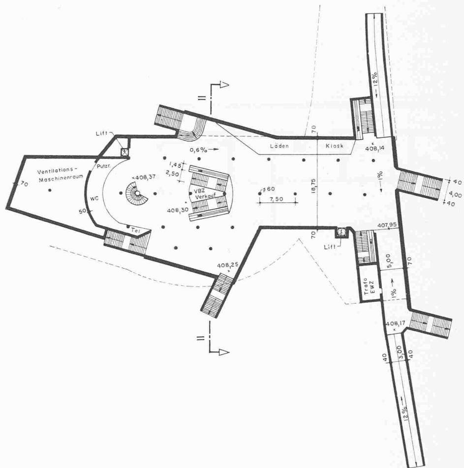
Bild 12. Fussgängerebene der Station Sihlporte, Grundriss 1:800. Schnitt 11 siehe Seite 853
