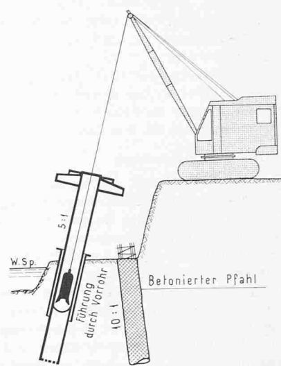
Bild 8. HW-Schrägpfählen an einem Steilufer
