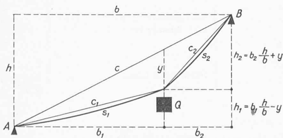
Bild 1. Lastfeld: Sehnennzug c_1 + c_2 und Last-Länge s_1 + s_2 des Tragseiles (Zugseil nicht eingezeichnet)
