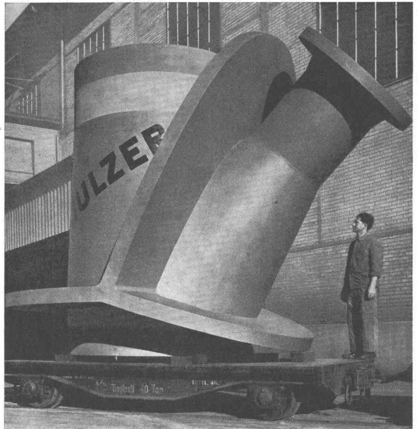
Eines der Abzweigrohre mit Sulzer-Verstärkungskragen der Verteilung Lünensee
