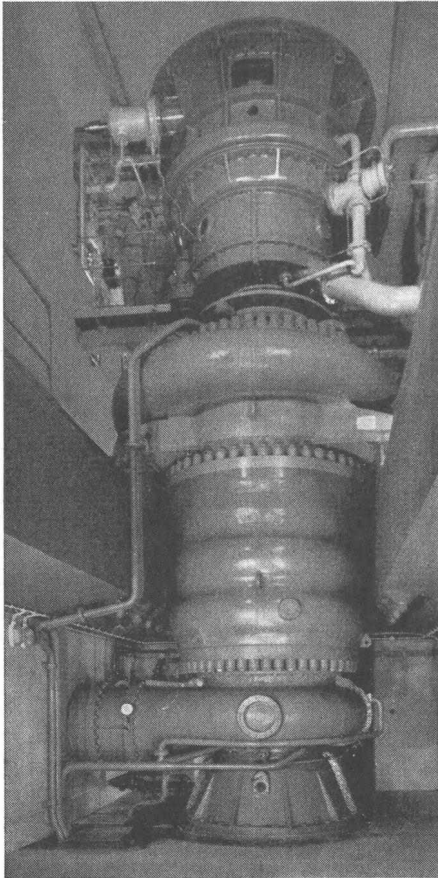
Sulzer-Hochdruck- Speicherpumpe im Kraftwerk Lünensee
