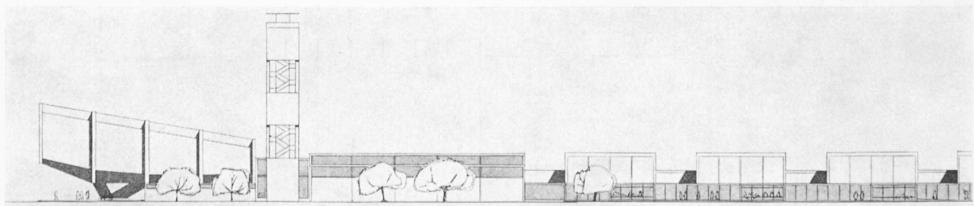
Strassenfassade 1:1000
