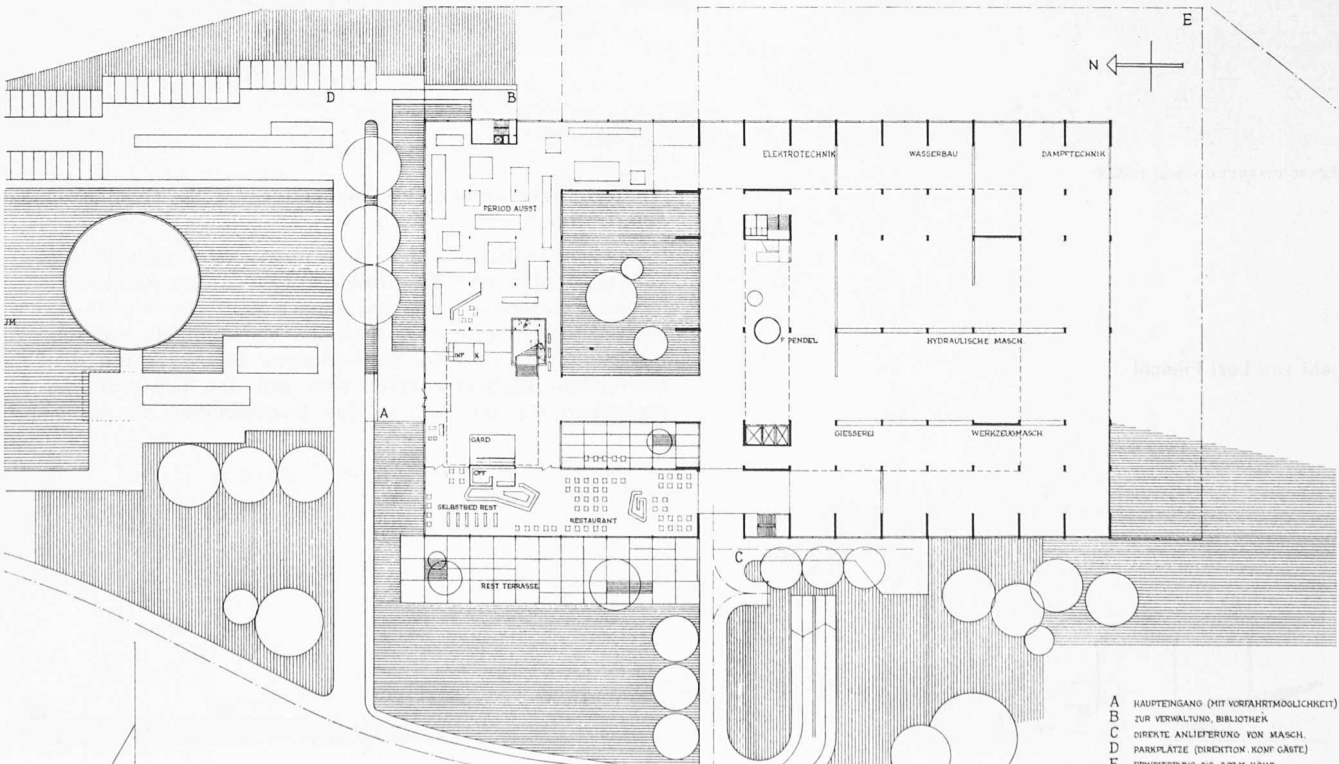
Erdgeschossgrundriss 1:1500
