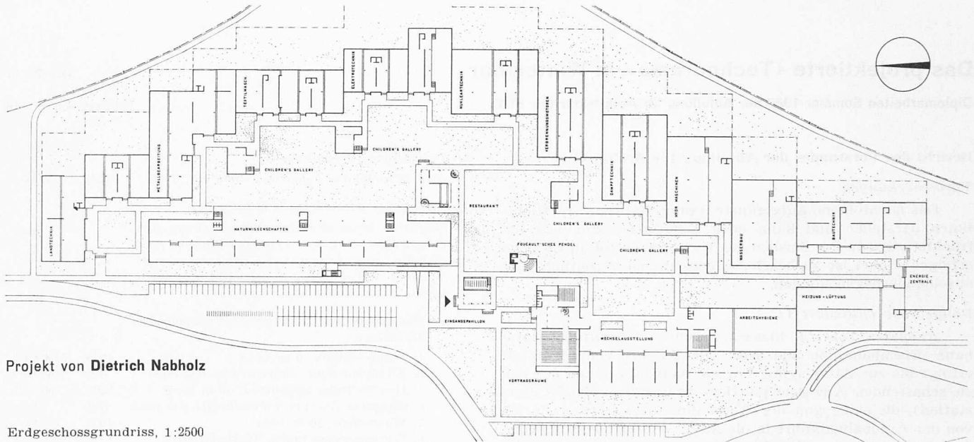
Erdgeschossgrundriss, 1:2500
