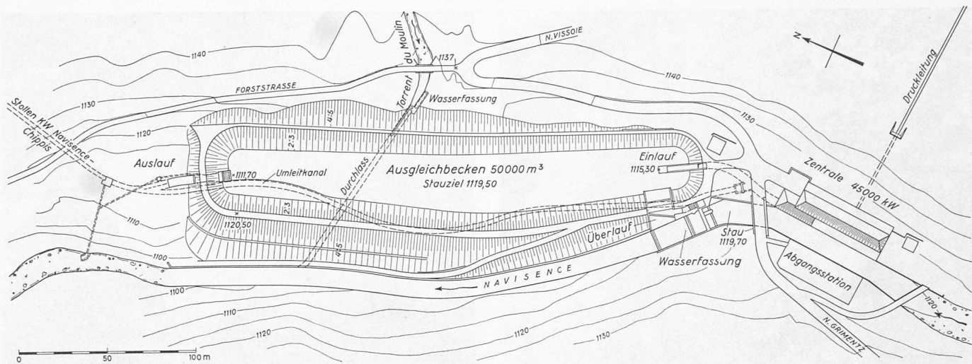
Bild 4. Ausgleichbecken Vissoie der Kraftwerke Gougra AG., Lageplan 1:3000
