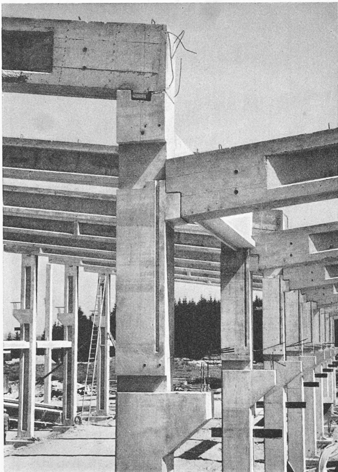
Bild 23. Details einer vorfabrizierten Halle der Stug in Zollikofen BE
