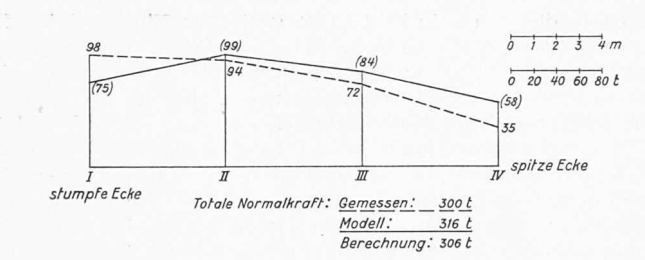
Bild 11. Querverteilung der Hauptmomente und Normalkräfte
