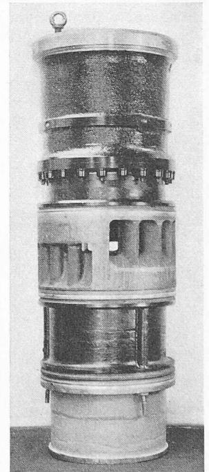
Bild 3. Ansicht des Zylindereinsatzes. Links die Spülschlitze, rechts die Auspuffschlitze
