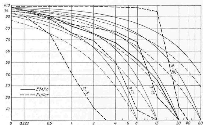
Bild 3. Siebkurven des verwendeten Baryt und seiner Komponenten
