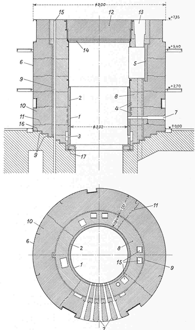
Bild 2. Vertikalschnitt (oben) und Horizontalschnitt (unten) durch den Reaktorschutzmantel, 1:150
