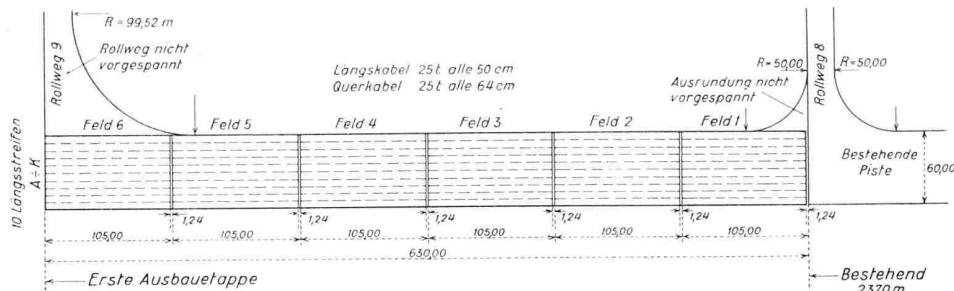
Bild 9. Flughafen Basel-Mülhausen, Vorschlag einer vorgespannten Piste, Masstab 1:6000
