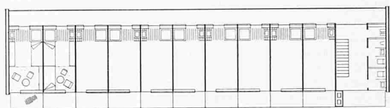
Gemeinschaftshaus Obergeschoss, 1:400
