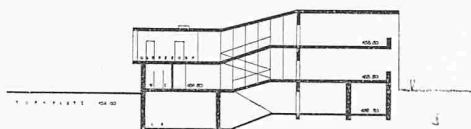
Schnitt Schulhaus
