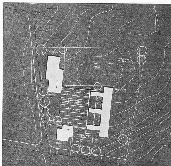
Lageplan 1:200
