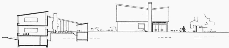
Schnitt Schulhaus
