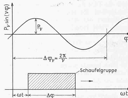
Bild 3 (rechts). Zur Berechnung von \alpha_\nu für eine Gruppe von grosser Schaufelzahl
