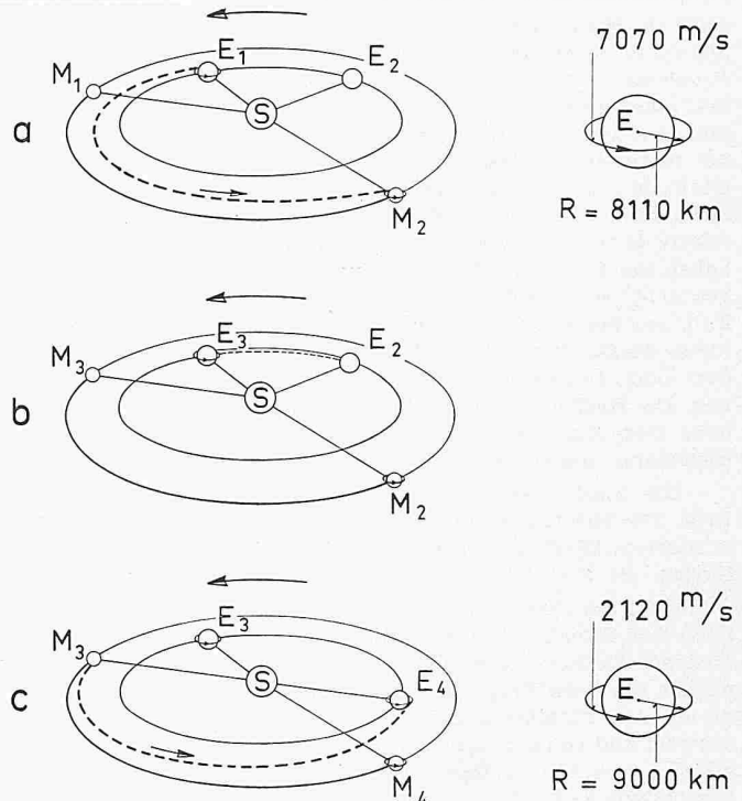
Bild 13. Mars-Expedition nach dem Projekt v. Braun . Ausgang von einer Erdsatellitenbahn. 260 Tage Ueberfahrt auf einer Kepler-Ellipse. Aufenthalt 449 Tage in einer Mars-Satellitenbahn. 260 Tage Rückreise und Einfang in eine (höhere) Erdsatellitenbahn. Für jedes einzelne Manöver sind rund 2 km/s Geschwindigkeitsänderung erforderlich. Während den 449 Tagen soll mit besonderen Raumschiffen (mit Tragflügeln) die Marsoberfläche besucht werden.
