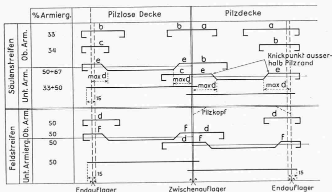
Bild 6. Anordnung der Armierungseisen Eisenlängen, gemessen von Auflagemitte:
