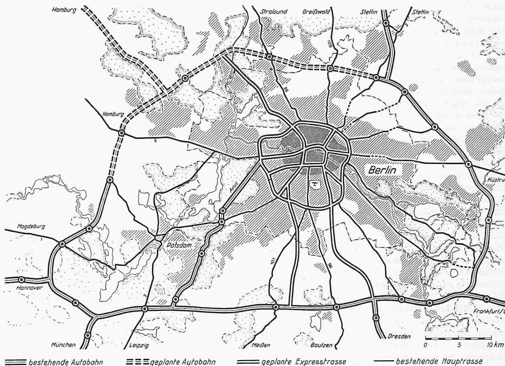
Bild 3 (rechts). Geplantes Expresstrassennetz in Berlin
