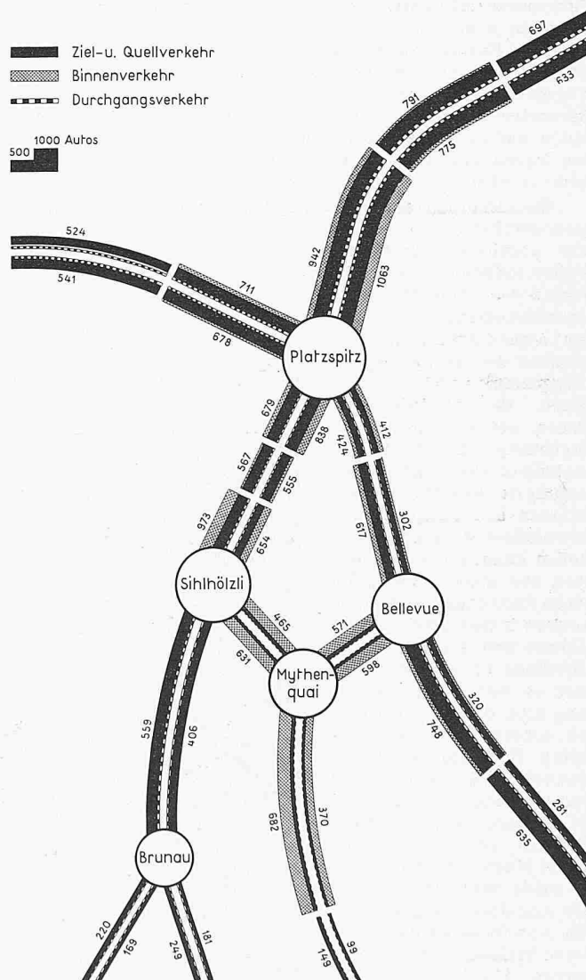
Bild 7. Belastungsplan (Autos pro Stunde) der Expresstrassen der Stadt Zürich auf Grund der Zählung vom 11. Juli 1955, 17.30 bis 18.30 Uhr
