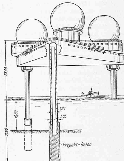
Schema des Aufbaues der Radarstation im Atlantik
