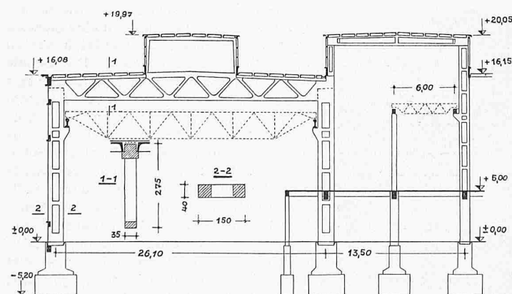
Bild 8. Graugiesereihalle, Querschnitt 1:500
