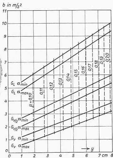
Bild 10. Verzugung als Funktion der Einfederung der Pufferfeder bei verschiedenen Belastungsfällen
