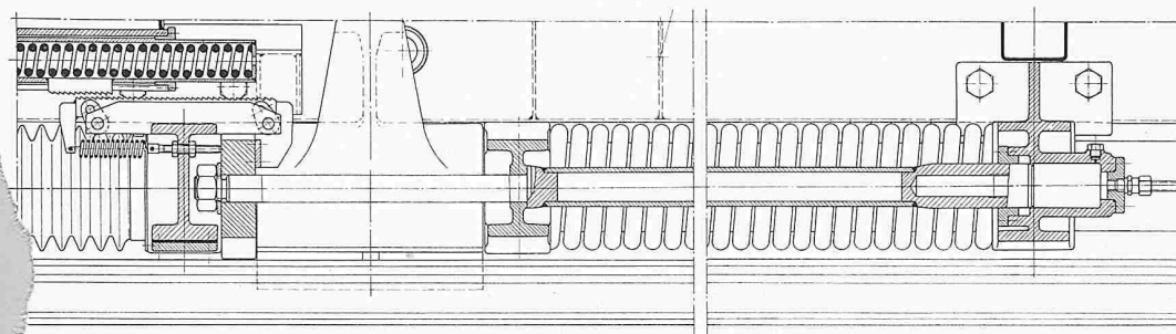
Längsschnitt C-C
