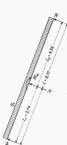
Bild 6. Zur Berechnung der Diagonalen a
