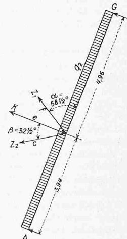
Bild 7. Schneedruck und Kräfte an der Diagonalen b
