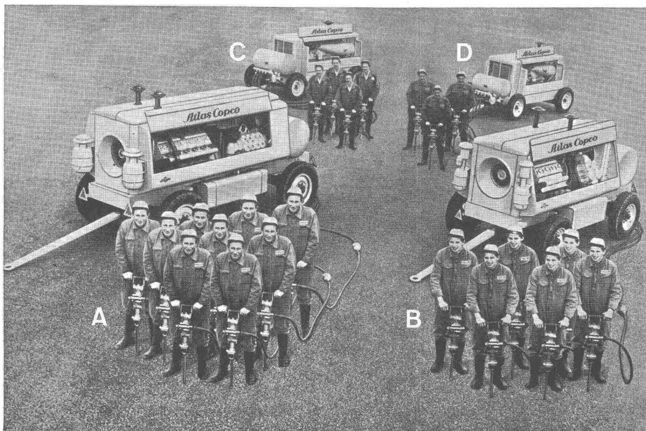
A Atlas-Copco, Typ 500 Dd, luftgekühlter zweistufiger Kompressor mit luftgekühltem 12-Zylinder-«Deutz»-Dieselmotor. Treibt bis zu 9 Bohrhämmer an.
