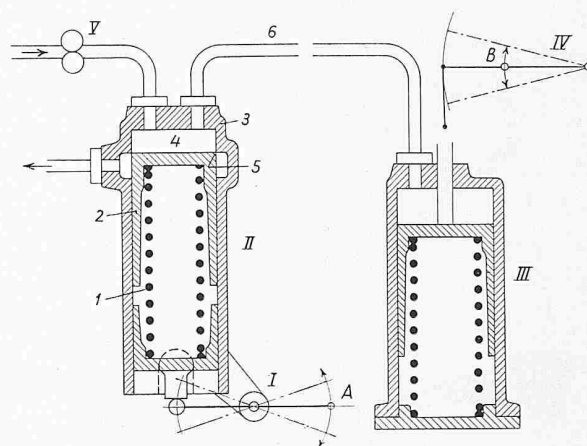
Bild 18. Schema der hydraulischen Rückführung, System Bell. Bezeichnungen im Text, S. 593
