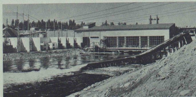
Bild 8. Kraftwerk von Unterwasserseite; rechts Flössrinne, links Schaltanlage
