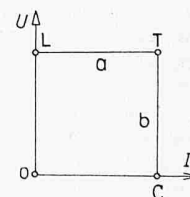
Bild 21. Regelung auf konstante Spannung (Ast a) und auf konstanten Strom (Ast b)
