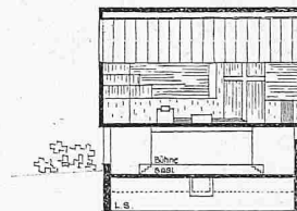
Querschnitt Holzwände in der Kirche Kanzelwand in vier Holzarten als flaches Relief ausgebildet
