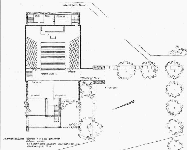
Kirchengeschoss, normal und mit Erweiterung (oben)
