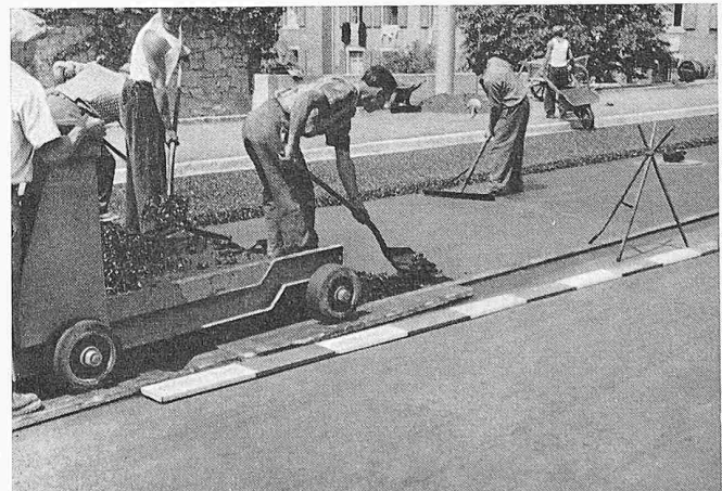
Bild 40. Einbau des Non-Skid-Belages auf der Grossbasler Zufahrtsrampe
