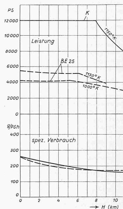
Bild 1. Vergleich von Leistung und spezifischem Brennstoffverbrauch des grossen Propellerturbinen-Luftstrahl-Triebwerkes PTL (Typenbezeichnung K, ausgezogen) mit dem modernen englischen Zweiwellentriebwerk B. E. 25 der Bristolwerke (gestrichelt) in Funktion der Flughöhe H
