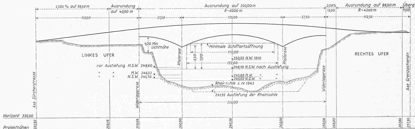
Bild 8. Längsprofil 1:3000/1:600 (fünffache Ueberhöhung) mit dem im Hinblick auf die Rheinschiffahrt einzuhaltenden freien Durchfahrtsprofil in der Mittelöffnung. Die eingetragenen Wasserspiegel beziehen sich auf den Zustand nach Fertigstellung der zurzeit noch im Gang befindlichen Austiefung der Rheinsohle
