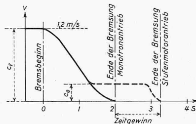
Bild 2. Verkürzung der Bremsdauer beim Monotronantrieb gegenüber einem Stufenmotorantrieb (Beispiel). Die Fahrgegeschwindigkeit von 1,2 m/s stellt für den Stufenmotorantrieb praktisch die obere Grenze dar, nicht aber für den Monotronantrieb
