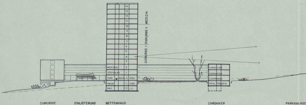
Querschnitt Bettenhaus, M. 1:1000
