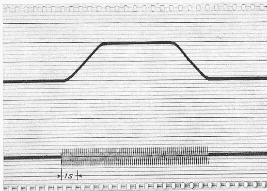
Bild 4. Ausschnitt aus einem Registrierdiagramm eines Monotronaufzuges. Oben Geschwindigkeitsverlauf. Man beachte die konstante Beschleunigung während der ersten Phase, bis die volle Fahrgegeschwindigkeit von rd. 1,5 m/s erreicht ist, sowie die konstante starke Verzögerung in der dritten Phase direkt bis zum Stillstand. Unten Zeitmarke, die durch die stärkere Schwingung den Zeitpunkt der Bremsöffnung und den der Bremserschliessung markiert. Diese erfolgt erst nach dem elektrischen Stillsetzen des Aufzuges.
