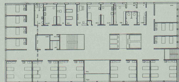
Südseite Chronikerabteilung, M. 1:1000
