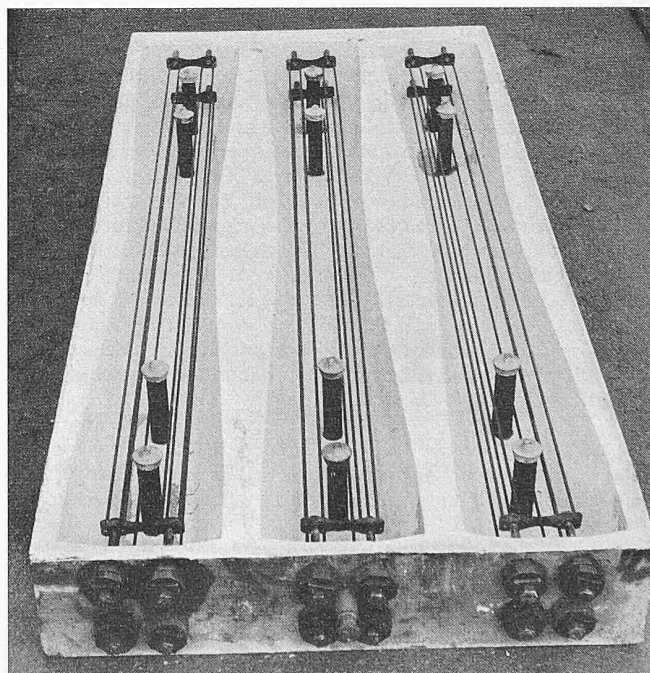
Bild 3. Vorspannarmierung System BBRV-Thosti
