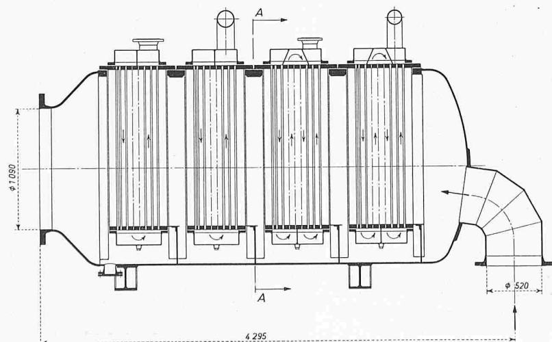
Bild 20. Längs- und Querschnitt durch den Vorkühler, 1:45
