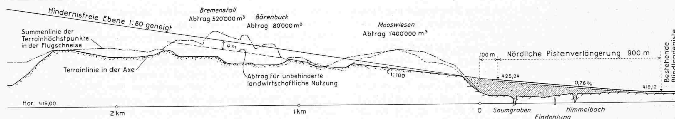
Bild 2. Längenprofil der Anflugschneise zur Blindlandepiste; Längensmasstab 1:20 000; Höhenmasstab 1:1600
