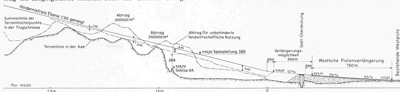
Bild 3. Längenprofil der Ausflugschneise von der Westpiste; Längensmasstab 1:20 000; Höhenmasstab 1:1600
