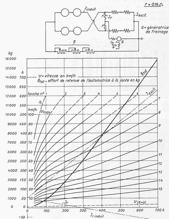
Fig. 9. Courbes caractéristiques du freinage à excitation séparée additive (mêmes moteurs qu'à la figure 8)
