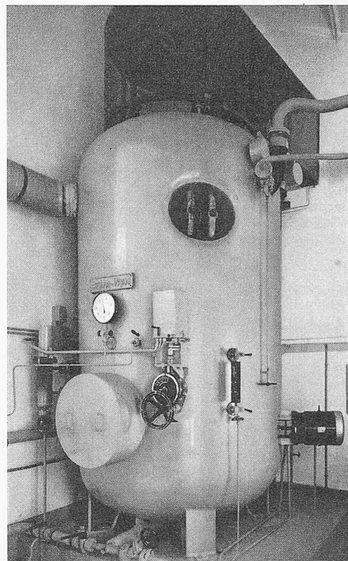
Bild 13 (rechts). Ansicht eines Escher Wyss Kaskaden-Elektrokessels, Leistung 3000 kW, Betriebsdruck 14 atü, Spannung 11 000 Volt
