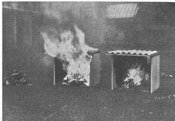
Das mit «ALBI-SKK» geschützte Dach hat sich nicht entflammt, obwohl die gleiche Menge Holz mit Benzin angezündet wurde. Aufnahme nach ca. 7 Minuten
