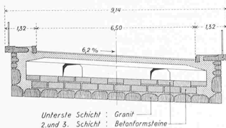
Bild 5 (links). Schnitt a-a im Scheitel; 1:150
